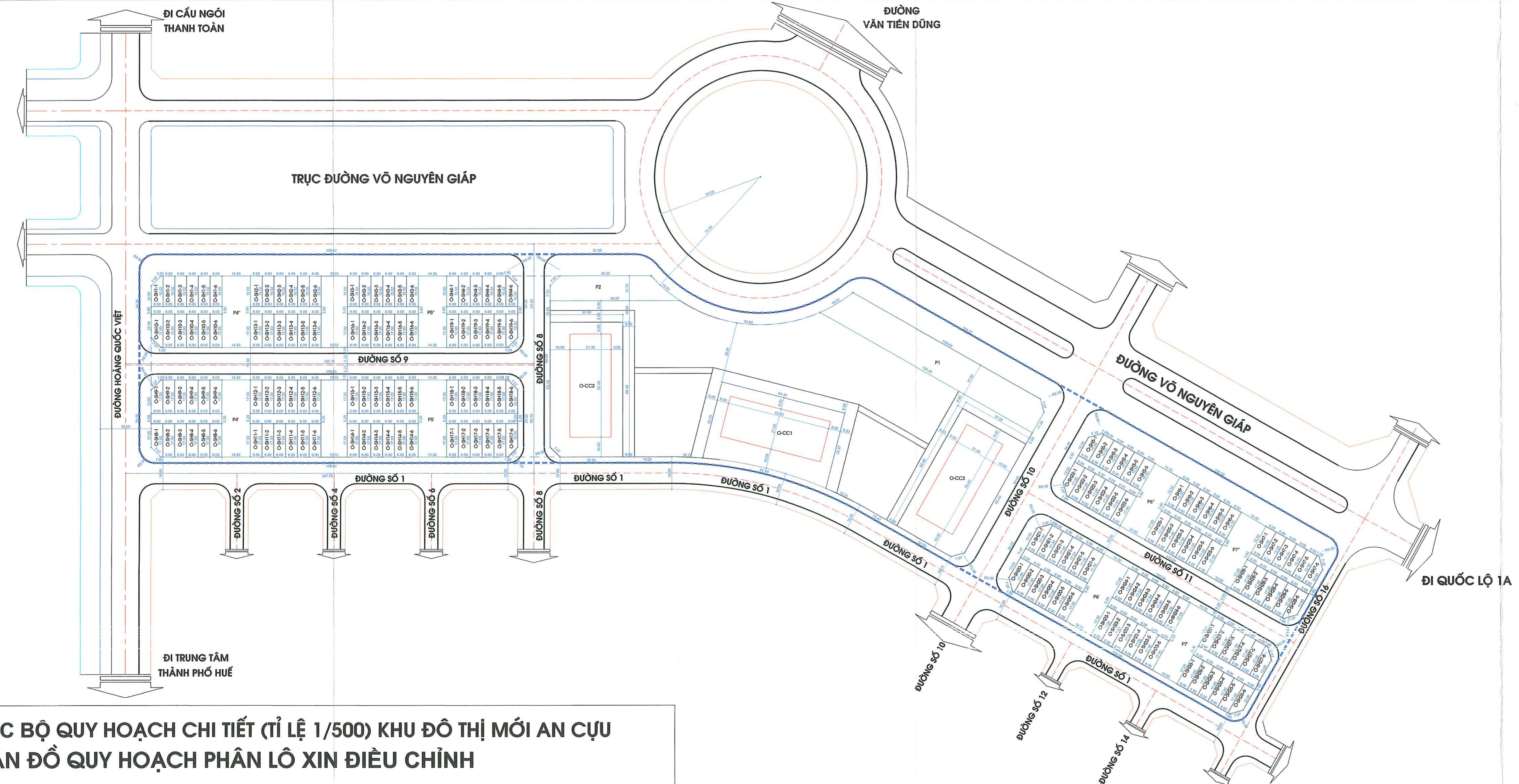
ĐIỀU CHỈNH QUY HOẠCH CHI TIẾT (TỈ LỆ 1/500) KHU ĐÔ THỊ MỚI AN CỤ BẢN ĐỒ QUY HOẠCH PHÂN LÔ ĐÃ PHÊ DUYỆT (QĐ/2932)
